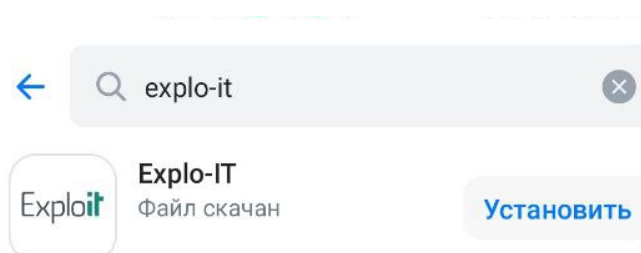
Рисунок 4. Установка приложения
